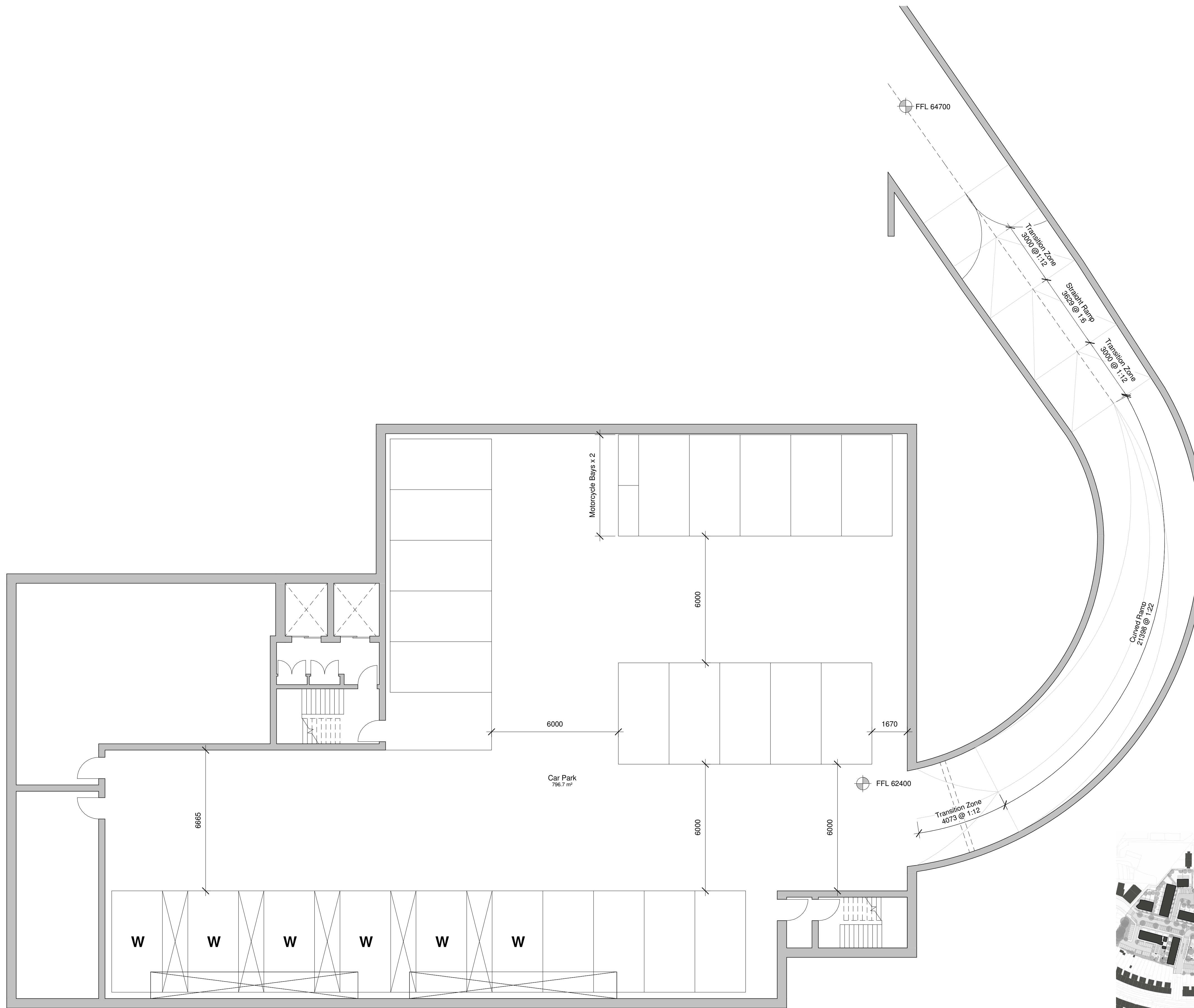
Block C - Basement Plan 1 : 100
